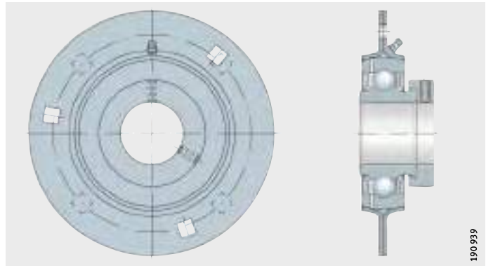
Figura 5 Soporte-brida, soporte de chapa de acero
